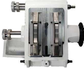
Gummer Unit
